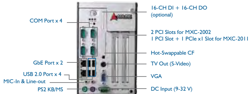
MXC-2002/MXC-2011 Front Panel
